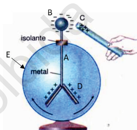
Fig. 12 - Electoscópio de folhas
