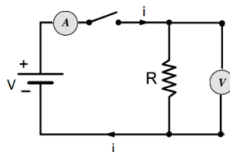
Fig. 36 - Circuito eléctrico
