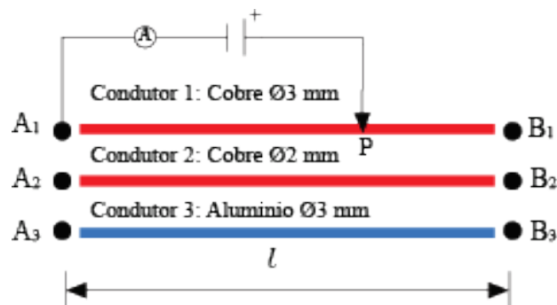
Fig. 41 – Resistência eléctrica de um condutor
