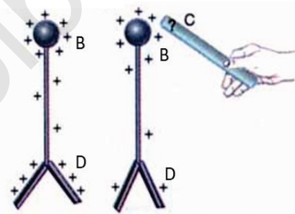
Fig. 14 - Determinação da carga eléctrica pelo electroscópio de folhas.
