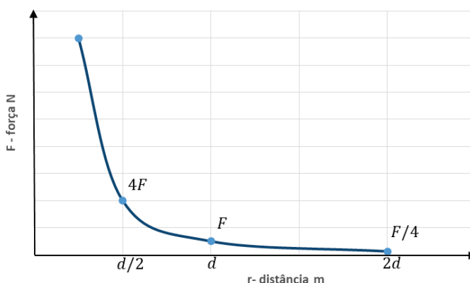
Fig. 17 - Gráfico da força electrostática em função da distância r
