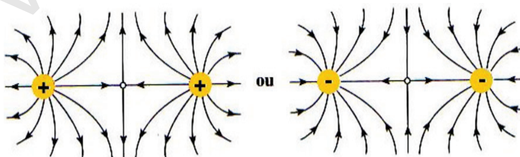
Fig. 21 - Campo eléctrico criado por duas cargas do mesmo sinal
