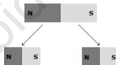
Fig. 43 - Leis qualitativas das interações magnéticas
