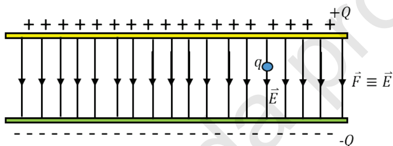
Fig. 23 - Campo eléctrico uniforme
