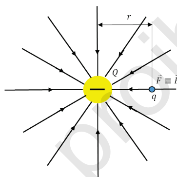
Fig. 20 - Campo eléctrico criado por uma carga negativa
