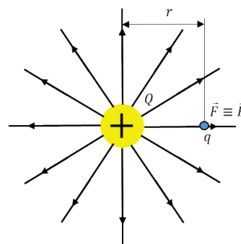
Fig. 19 - Campo eléctrico criado por uma carga positiva
