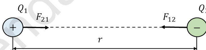
Fig. 16 - Força electrostática entre duas cargas
