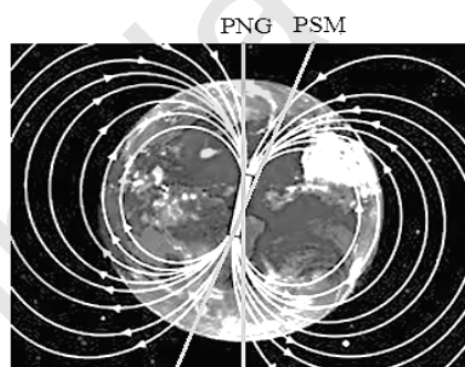
Fig. 46 - Linhas do campo magnético da terra, em que PNM é o pólo norte magnético, PSM, pólo sul magnético, PPSG, pólo norte geográfico e PSG, pólo sul geográfico.
