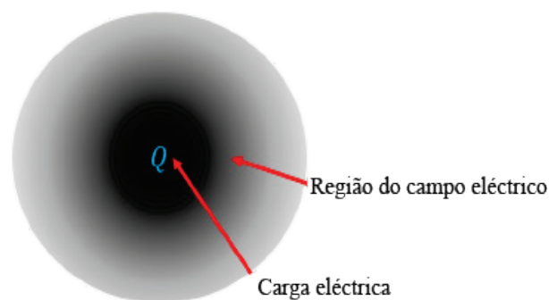
Fig. 18 - Região do campo eléctrico criado por uma carga
