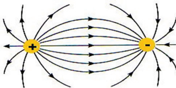
Fig. 22 - Campo eléctrico criado por cargas de sinais contrários
