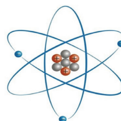
Fig. 1 - Átomo
